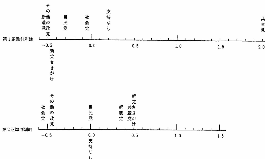
Fig. 1 各群の正準判別得点平均値のプロット
