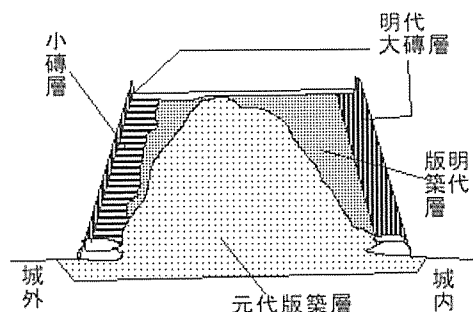
図6 北京内城壁断面略図
